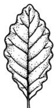
SINUATE
